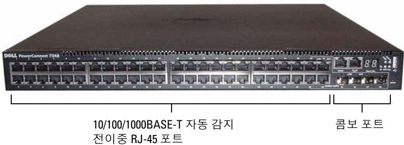
그림 1-4. 48개의 10/100/1000BASE-T 포트가 있는 PowerConnect 7048
